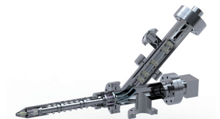
EQS SIMS Spectrometer
